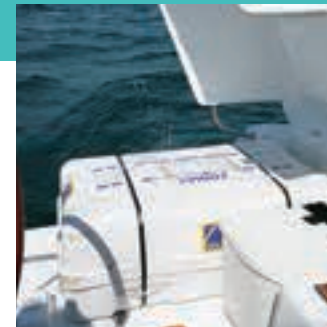
Coffre à BIB et à gaz avec ouverture assistée par vérin à gaz en inox • Liferaft and gas cylinder locker with stainless steel gas strut-assisted lid • Gavone zattera e per bombola gas con apertura assistita con attuatori in inox a gas • Cofre balsa salvavidas con abertura asistida por retenedor a gas inox • Backskiste für Rettungsinsel und Gasflasche mit Niro-Gaszylinder zum Öffnen
