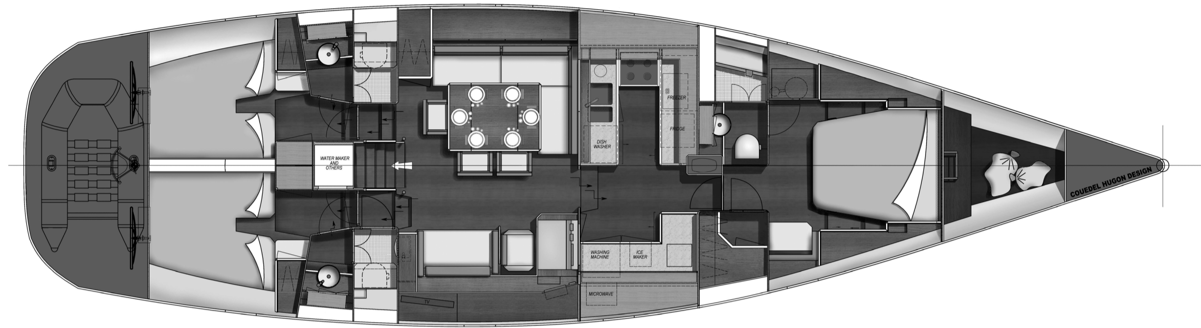
1. BORDEAUX 60 version propriétaire avant BORDEAUX 60 forward owner's cabin layout
