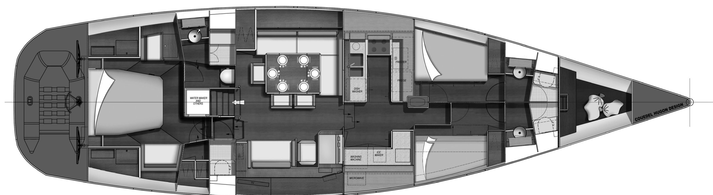
4. BORDEAUX 60 version propriétaire arrière BORDEAUX 60 aft owner's cabin layout
