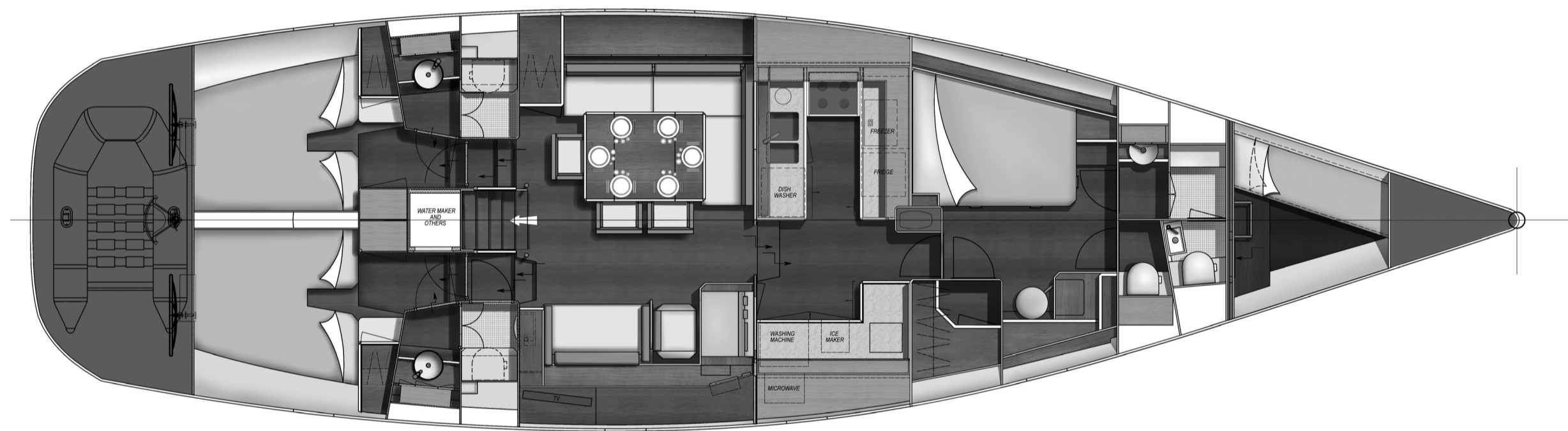
2. BORDEAUX 60 version propriétaire avant avec lit latéral et zone équipage BORDEAUX 60 forward owner's cabin layout with lateral bed + crew area
